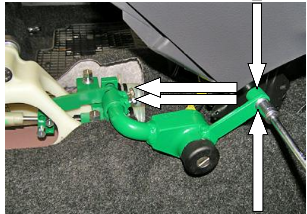
Установить замок, подложив столбик 15 мм. под лапку, закрутить болт, зафиксировать трубу замка в кольце детали-переходника
