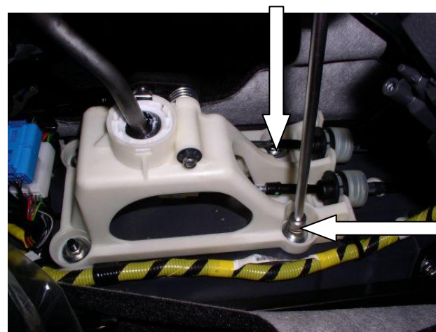
Открутить 2 гайки
