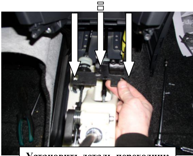
Установить деталь-переходник на столбики, закрутить 2 болта
