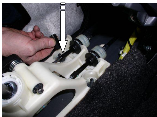
Установить шестигранный столбик на шпильку
