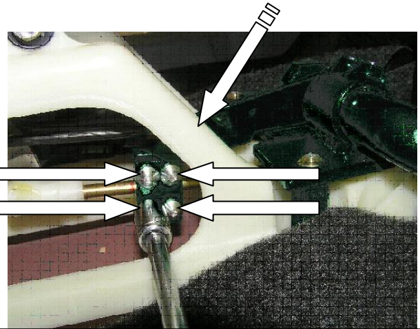
Установить хомут на тягу, зафиксировать
