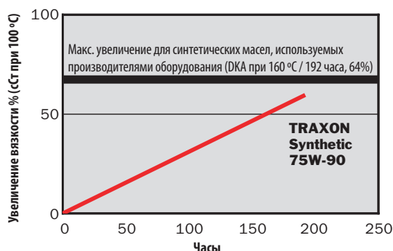
Испытание на окисляемость ДКА (CEC-L-48-A-95) (192 часа при 160 °C) GL-5 75W-90 Synthetic
