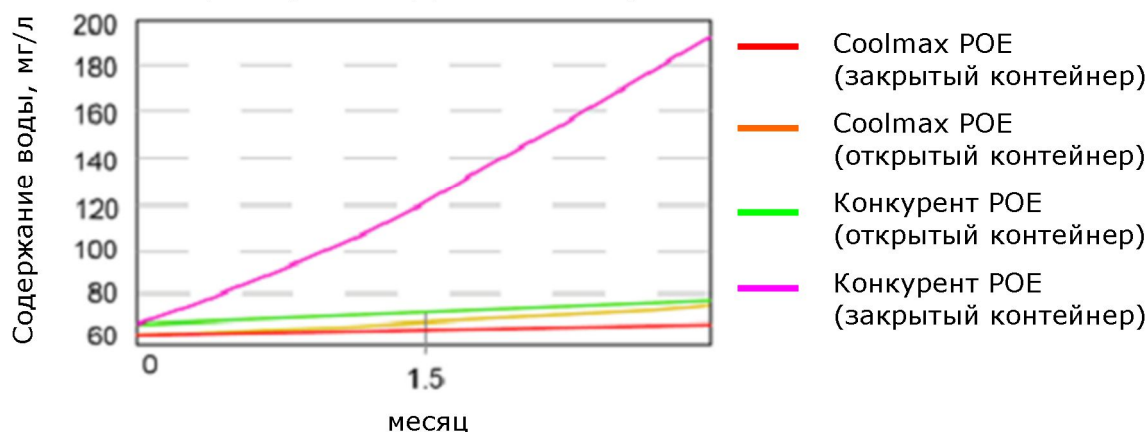
Количество абсорбированной воды (по Карл Фишеру ASTM D6304)
