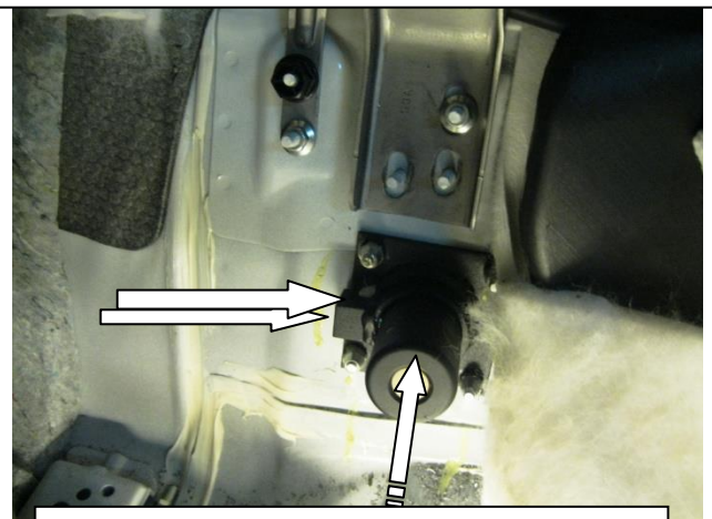
Установить прямоходный цилиндр в кронштейн замка, зафиксировать
