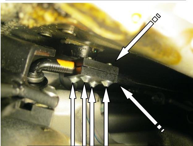
Установить хомут на тягу под днищем, зафиксировать
