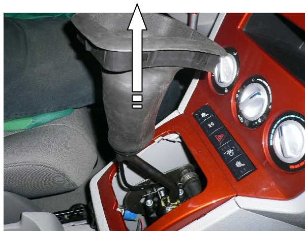
Снять декоративный кожух рычага переключения передач
