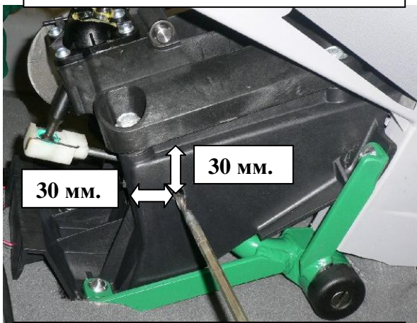
Просверлить технологическое отверстие в селекторе по разметке
