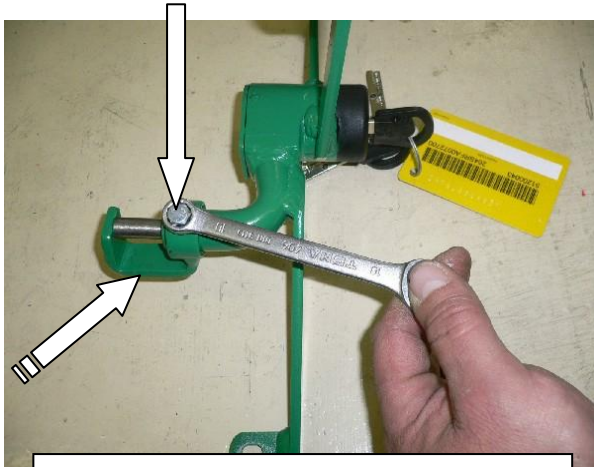
Установить защиту тяги на трубу замка, зафиксировать винтом
