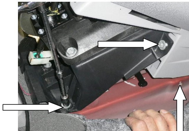
Открутить 3 болта
