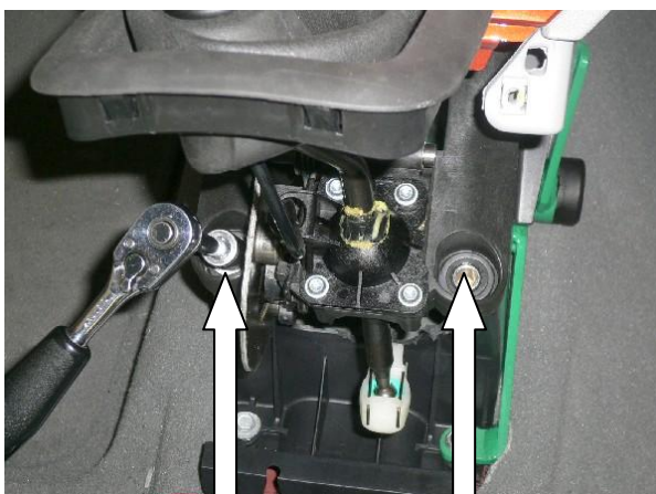
Открутить 2 штатных болта крепления селектора, заменить на срывные
