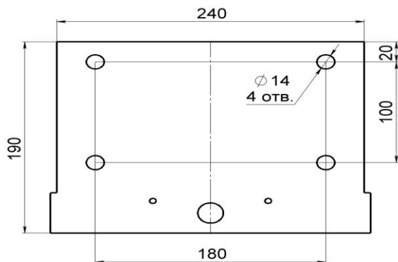
Рис 2 Шаблон сверления для стойки
