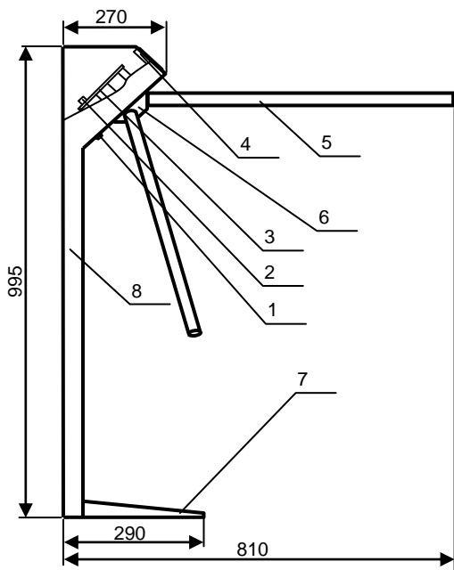
Рис. 1 Общий вид
