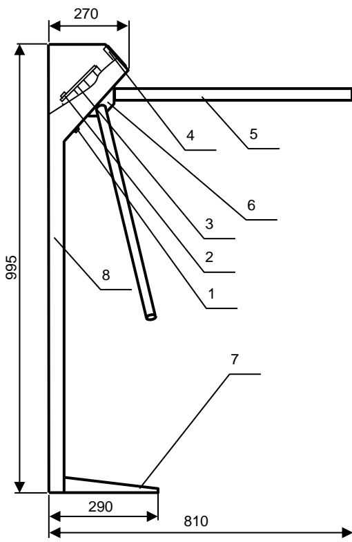
Рис. 1 Общий вид
