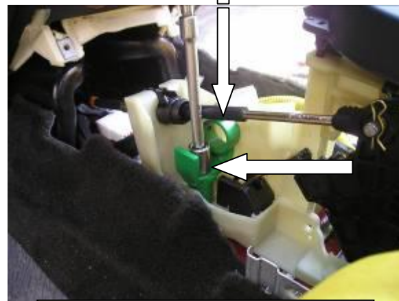
Установить кронштейн замка, закрутить срывной болт
