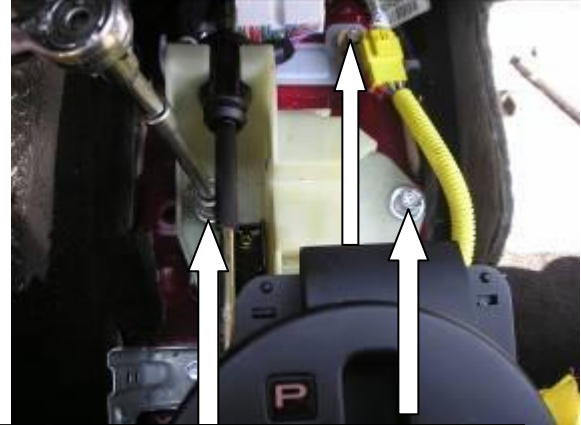
Открутить 3 штатных болта
