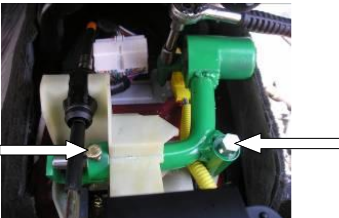
Установить замок на столбик, закрутить срывной болт, зафиксировать трубу замка в кольце кронштейна замка винтом
