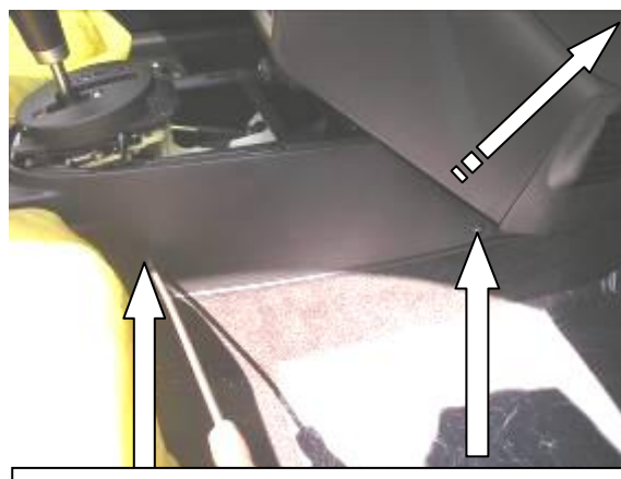
Поднять заднюю часть консоли, открутить саморезы с обеих сторон
