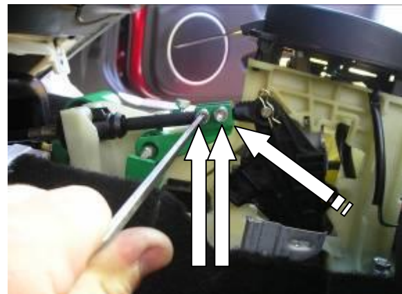
Установить хомут на тягу, зафиксировать 2 винтами, перевести рычаг переключения передач в положение «Р», произвести блокировку, отрегулировать положение хомута на тяге, сорвать винты
