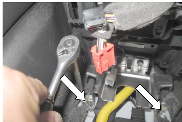
Открутите два болта крепления кронштейна
