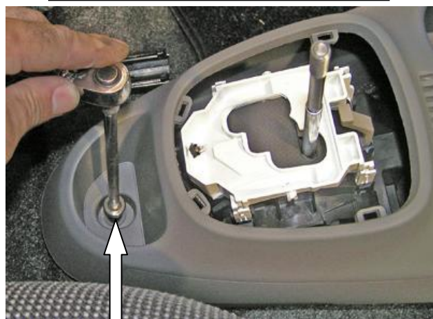
Открутить саморез
