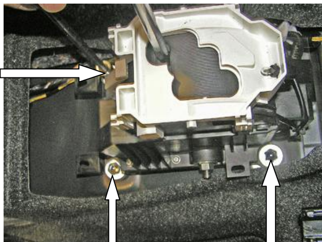
Открутить 3 болта
