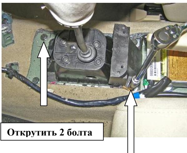
Снять переднюю консоль
