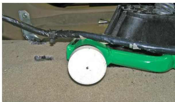
Разметить, используя разметочный шаблон, отверстие в консоли под корпус замка
